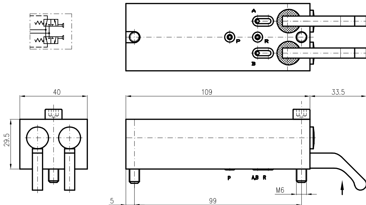
Abbildung: pm3/val/evv/h1 Handbetätigtes Vorsteuerventil
